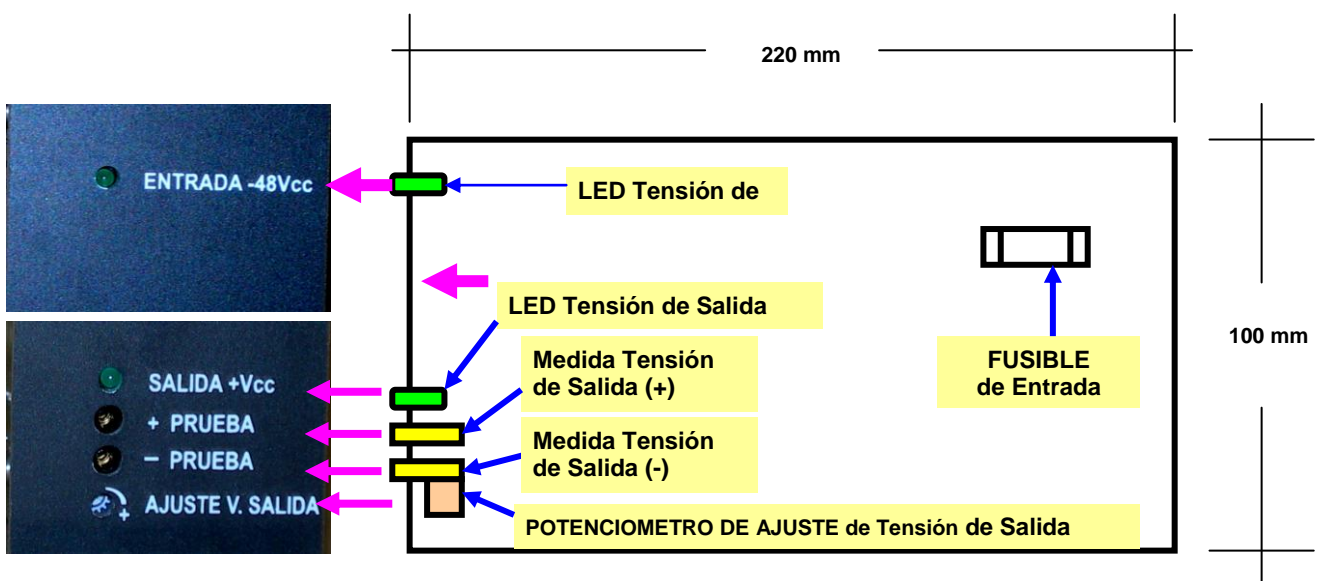
TARJETA DEL CONVERTIDOR DC/DC ENERTEL 48Vcc / 24Vcc - 280W : Dimensiones y Posicional de Componentes de Medida, Ajuste , Señalización y Protección
